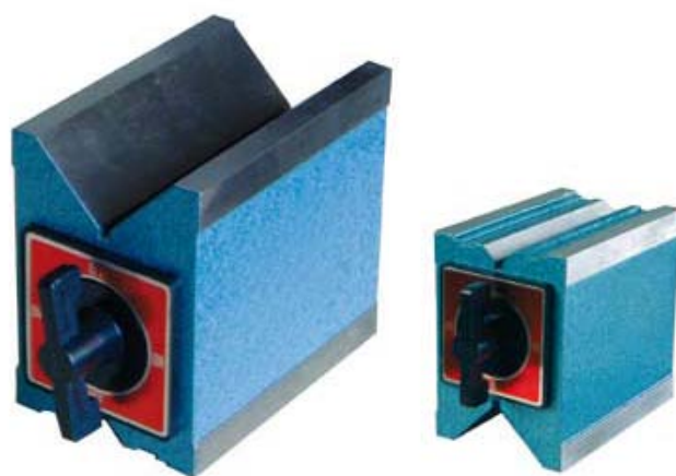
Art. 540/5 – Coppia di prismi magnetici di alta precisione toll. 0,01 Magnetic v-block pair, accuracy 0,01mm, hardened, with magnet, on and off switch, 90° grooves
