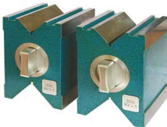
Art. 542 – Coppia di prismi magnetici di alta precisione toll. 0,005 Magnetic V-block pair, accuracy 0,005 mm, hardened, with magnet, on and off switch 90° grooves, 90° on the side, front end 90°, magnet force switchable
